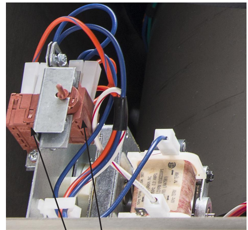
Thermoactuators
