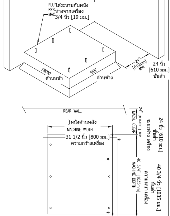
แผนผังพื้น ภาพที่ 1-2
